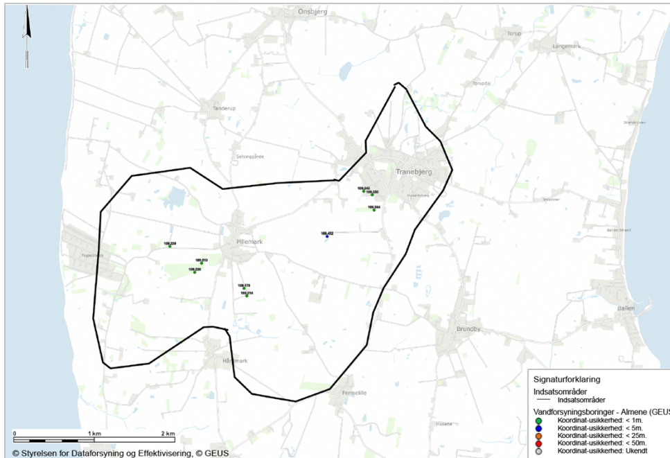
Figur 2.6. OSD og indvindingsboringer på Sydsamsø
